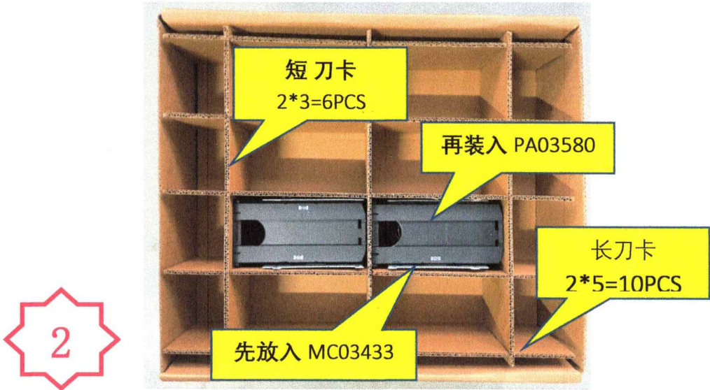
图二, 箱子底部先装一个隔板, 再将刀卡装好放入箱子, 1 层 8 格, 1 格装 1 个 PA03580+MC03433, 装满后盖上隔板, 一箱 2 层, 共 16 个。
